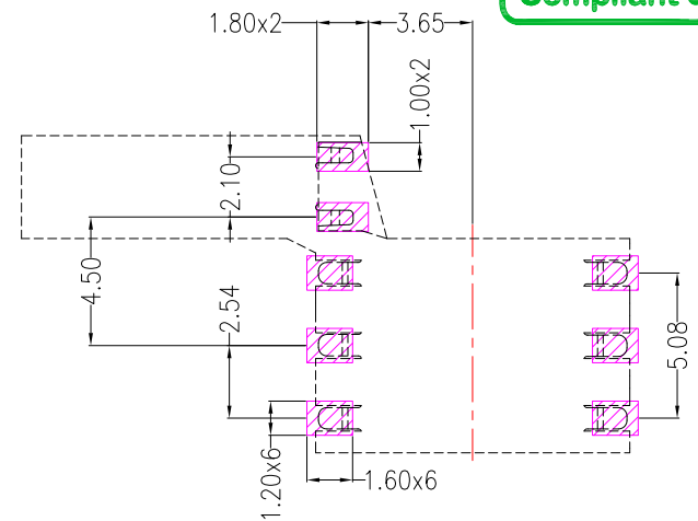
P.C.B Layout
