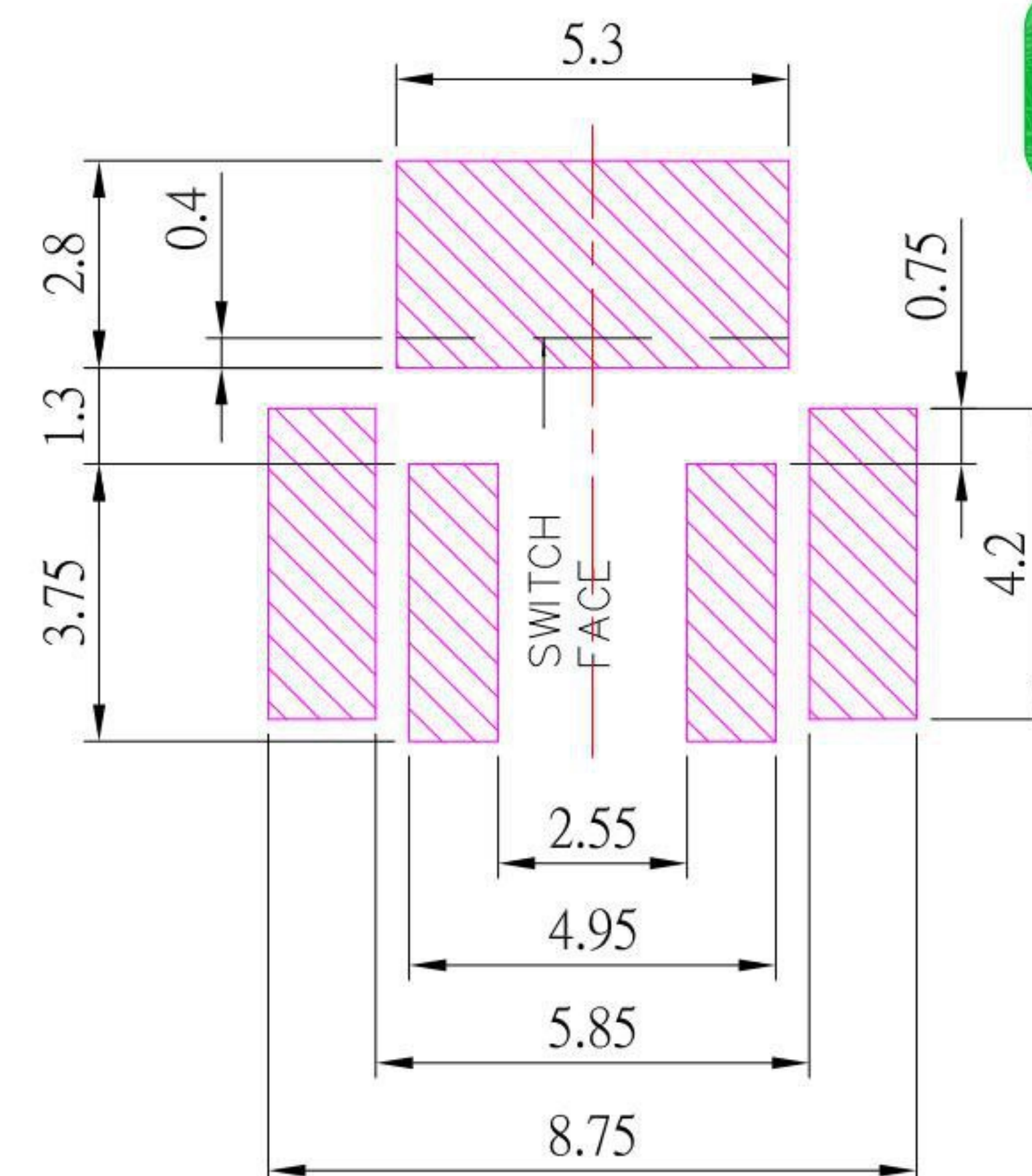
P.C.B LAYOUT
