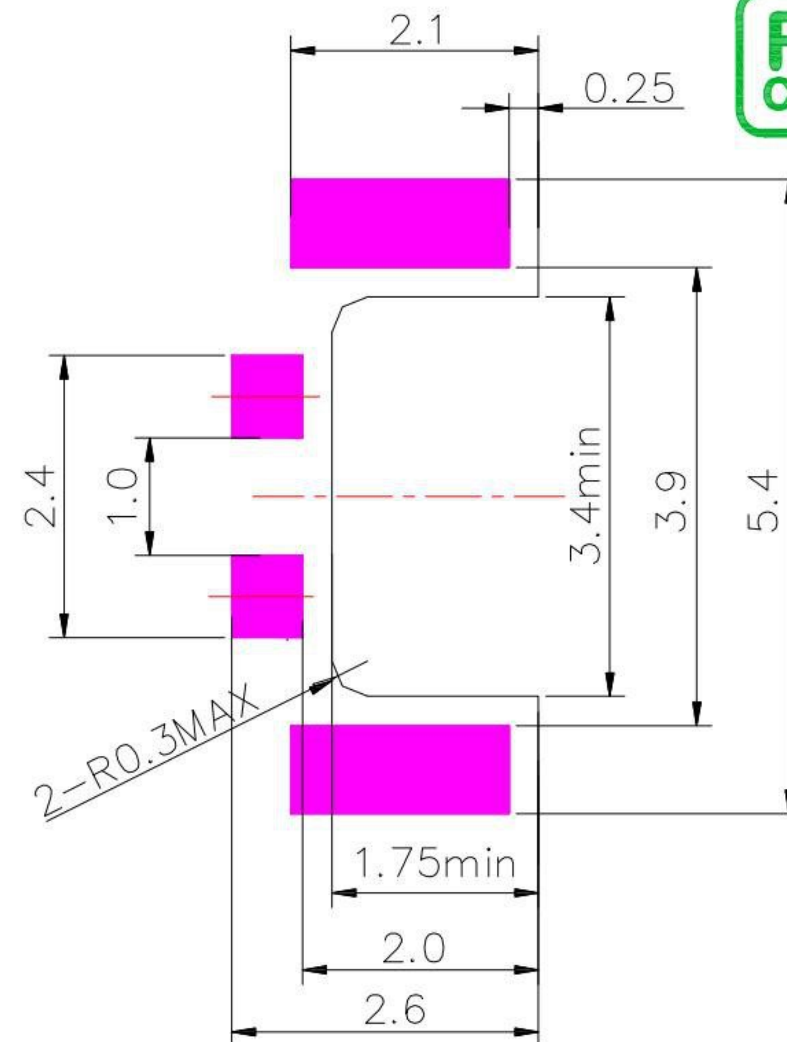
P.C.B LAYOUT
