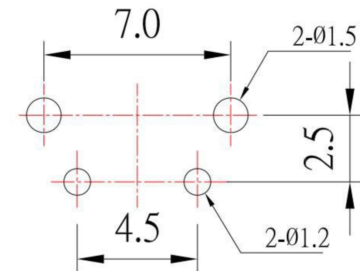
P.C.B LAYOUT
