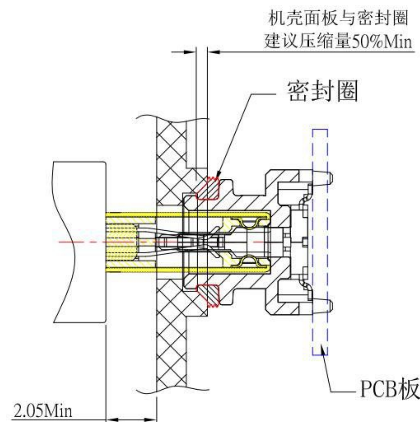
组装面板后公母头对插示意图
